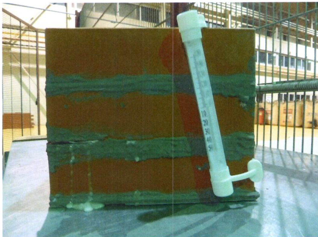
Рис.2.1. Фрагмент кладки №1
